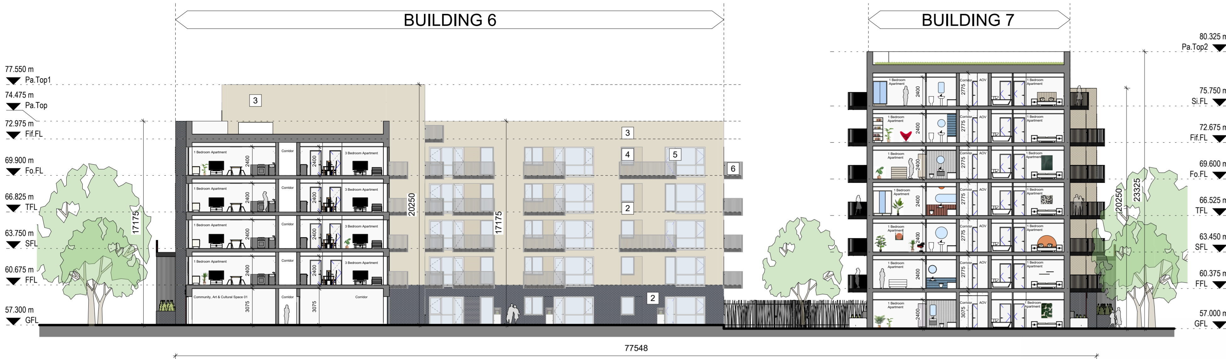
1 Section A-A 1 : 200
